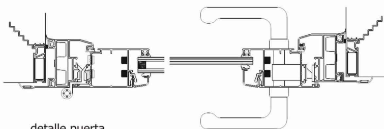
detalle puerta
